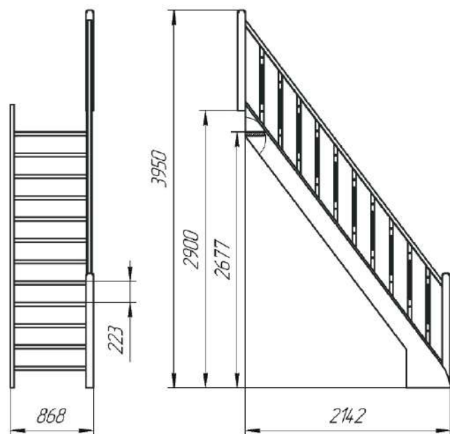
Рисунок 1. Лестница внутриквартирная ЛЕС-12.
